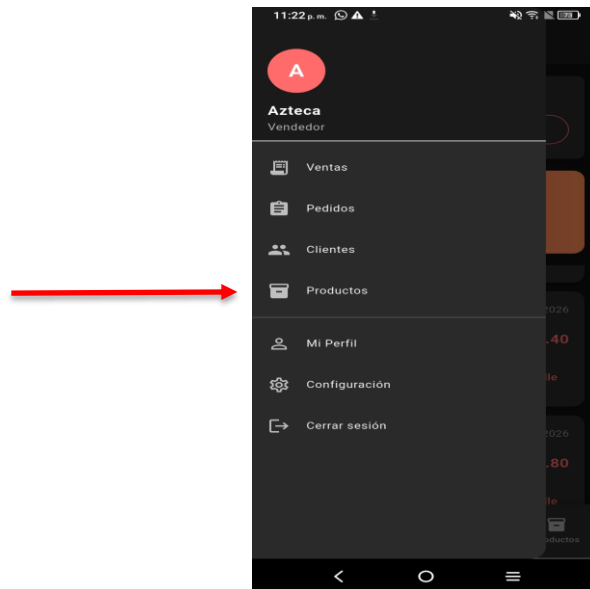
Ilustración 97. Menú Principal de Navegación.
