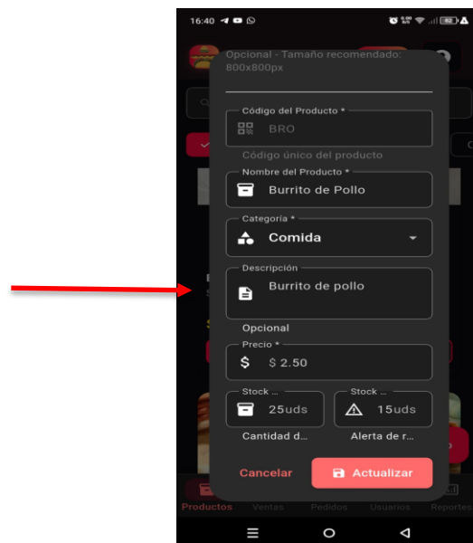
Ilustración 114. Pantalla de Edición y Actualización de Producto Existente.
