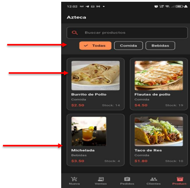
Ilustración 95. Pantalla de Productos del Vendedor.
