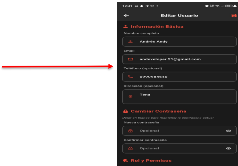
Ilustración 122. Pantalla de Edición de Usuario
